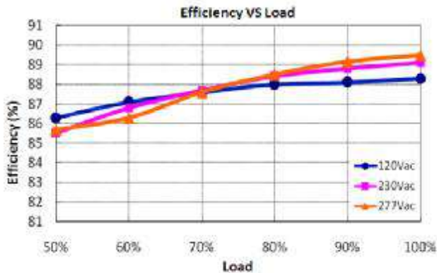
X6-075Y062 (Io=1.21A)
