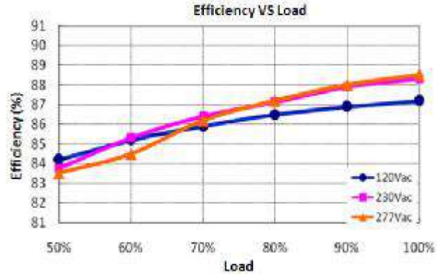
X6-075Y062 (Io=1.88A)
